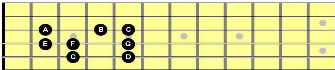
C-Dur Tonleiter
