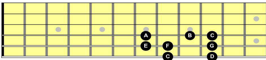
C-Dur Tonleiter
