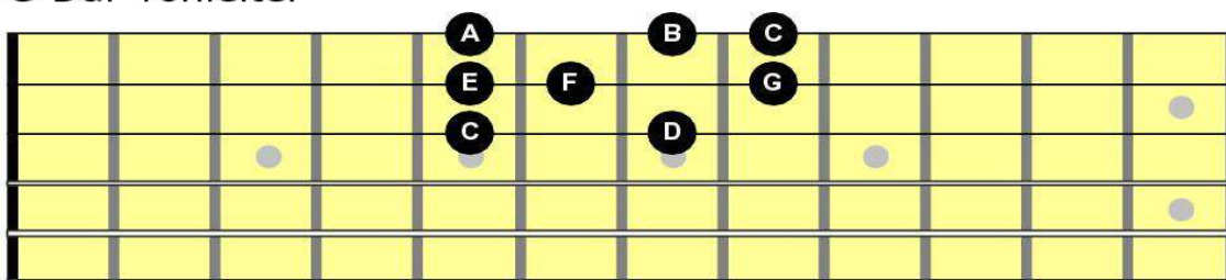
C-Dur Tonleiter
