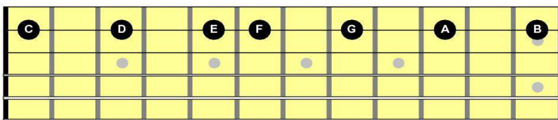
C-Dur Tonleiter
